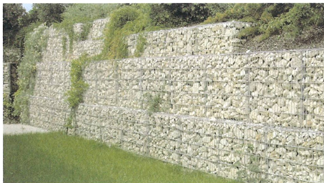
Bewachsen garantieren Gabionen eine naturnahes Erscheinungsbild
